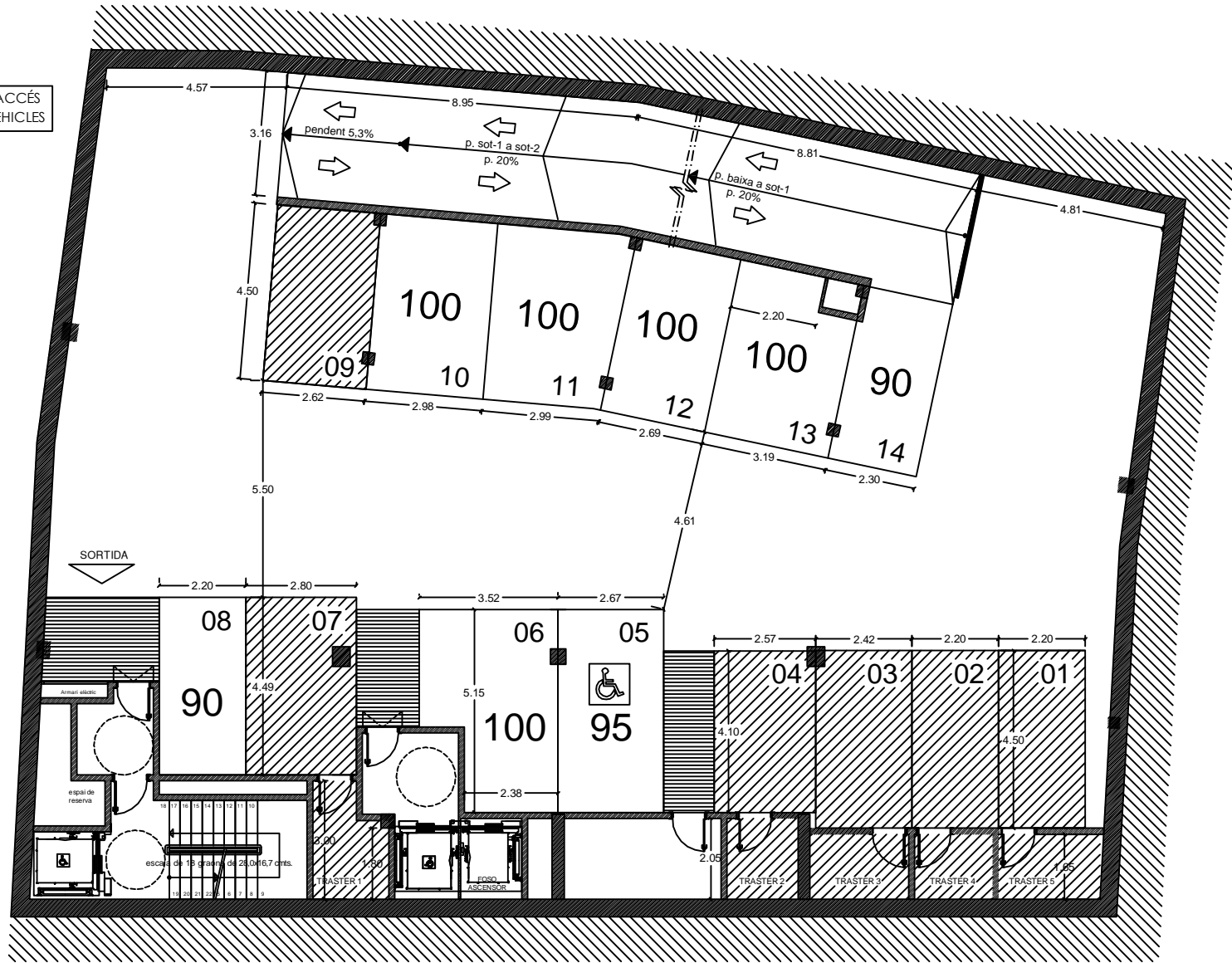
PLANTA SOTERRANI -1
